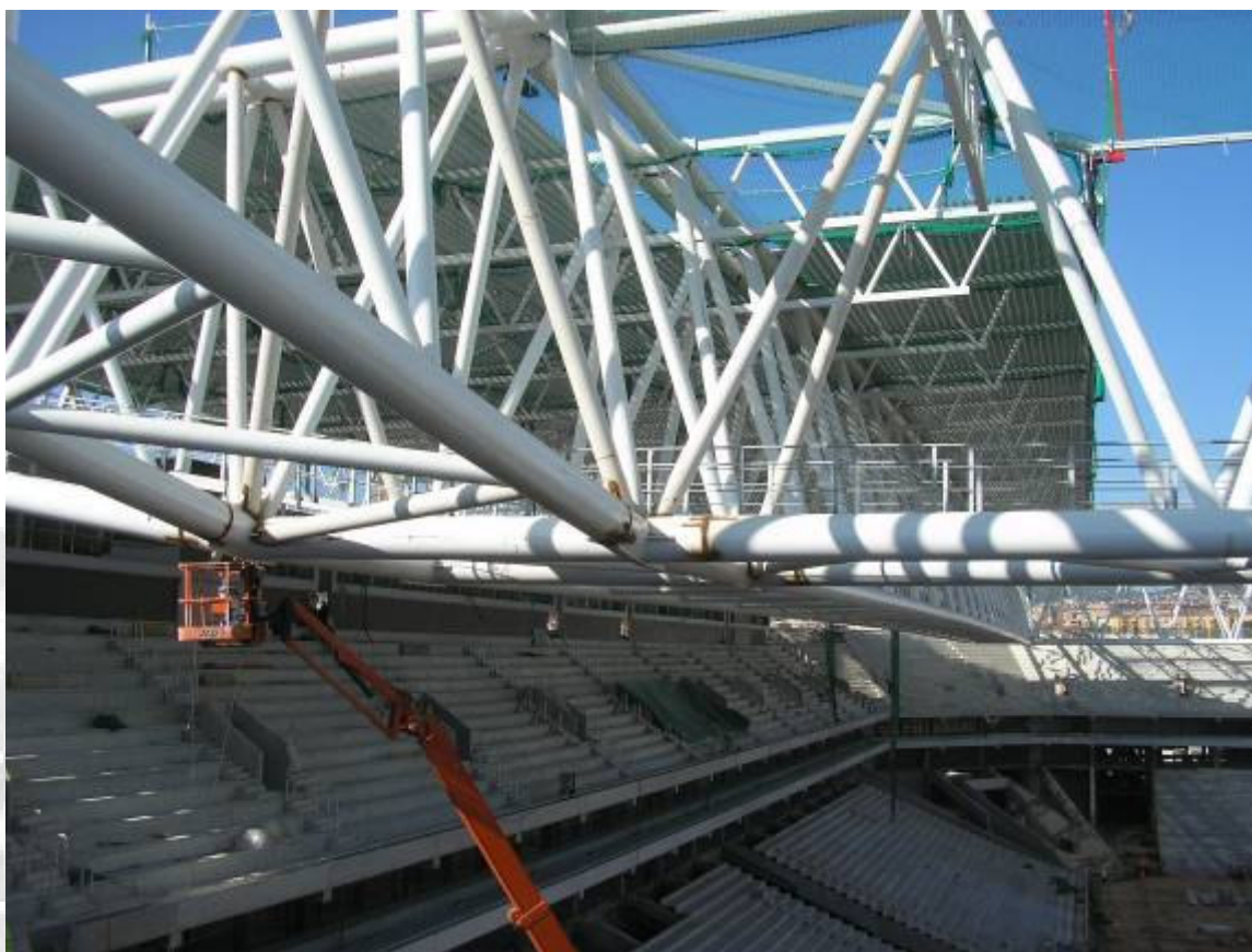
Vista de les xarxes horitzontals sota encavallades de la coberta i perímetre de xarxa tipus tennis de 2,00 m d'alçada (en anell interior i exterior de la coberta) per al muntatge de xapes de coberta de l'estadi.
